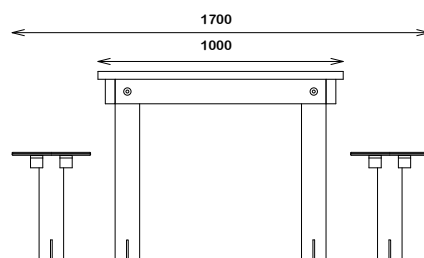
627 939-01 table de jeux - damier étoile mesa de juego - tablero estrella play table - stella game
